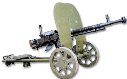
12,7-мм крупнокалиберный пулемет Дегтярева — Шпагина
